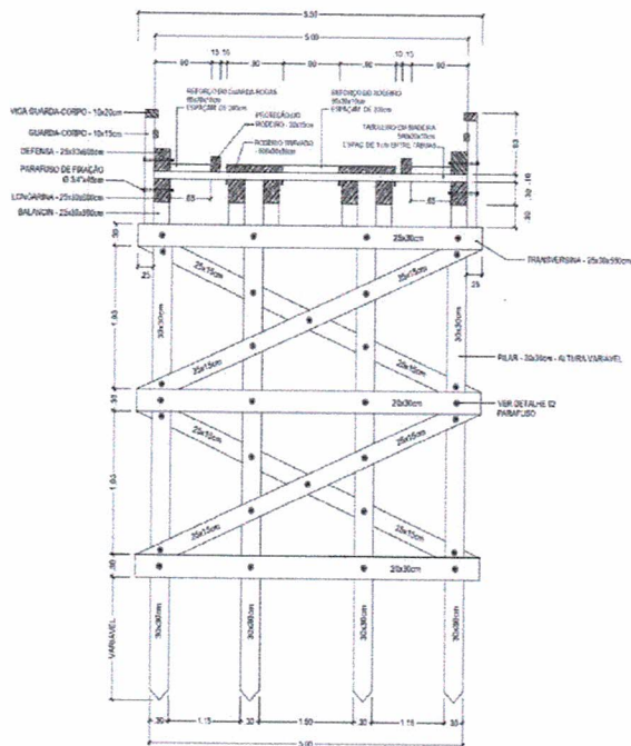
Seção Transversal da Ponte S/Escala
